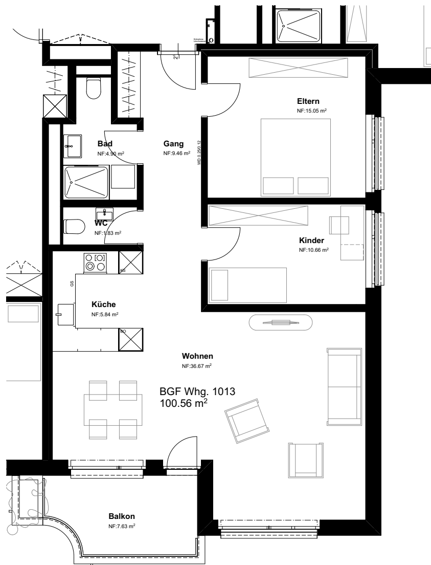
Grundriss 3 1/2 Wohnung 1:100
